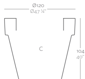
Maceta Ø47 ¼" Maceta Ø120 cm
