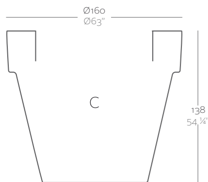
Maceta Ø62" Maceta Ø160 cm
