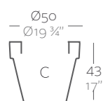
Maceta Ø19 ¾" Maceta Ø45 cm
