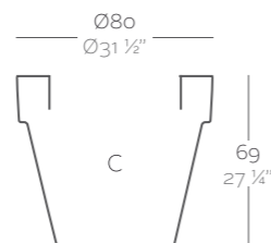
Maceta Ø31 ½" Maceta Ø80 cm
