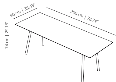
MAA200_ table 200x90 | 35 7 / 16 x 78 47 / 64
