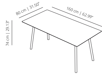
MAA160_ table 160x80 | 31 1 / 2 x 62 63 / 64
