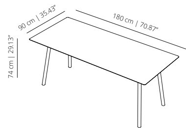
MAA180_ table 180x90 | 35 7 / 16 x 62 63 / 64
