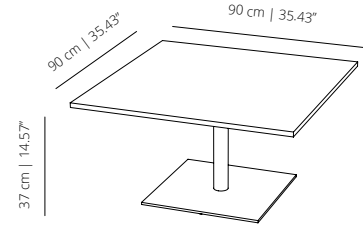
ST37C90_ table 90x90 | table 35 7/16 x 35 7/16
