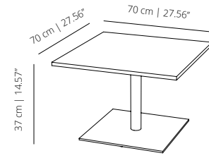
ST37C70_ table 70x70 | table 27 6/16 x 27 6/16
