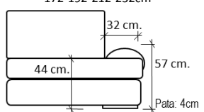
1 brazo / 1 Arm 92-102-112-122-152-172-192-212-232cm
