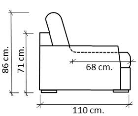
1 brazo / 1 Arm 92-102-112-122-152-172-192-212-232cm
