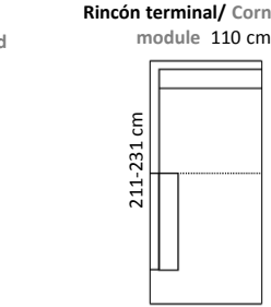
Rincón/ Corner 110 cm
