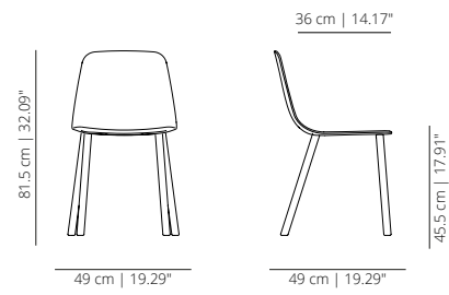
MAAPL4PM plastic
