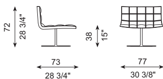
REF. 434-SCG Base cuadrada y giratoria Square base / swivel
