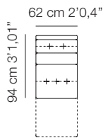
Módulo 62 Fijo Módulo 62 Relax Ref. 105726 Ref. 105727
