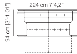
Sofá 4 Plazas Fijo Sofá 4 Plazas 2 Relax Ref. 105741 Ref. 105740
