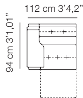
Módulo 87 C/B Fijo BD 105742 BI 105743
