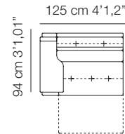
Módulo 100 C/B Fijo BD 105764 BI 105765
